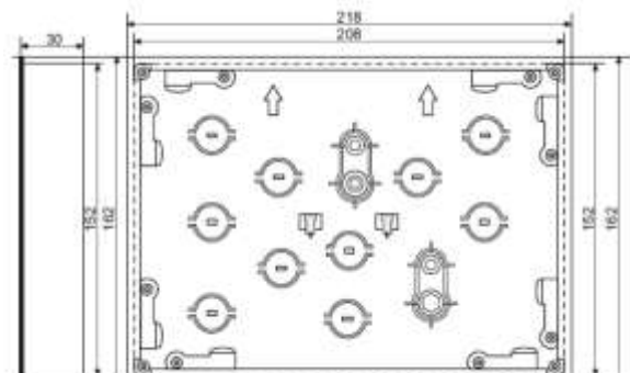
Размеры металлической коробки для монтажа клавиатур на кирпичную стену
