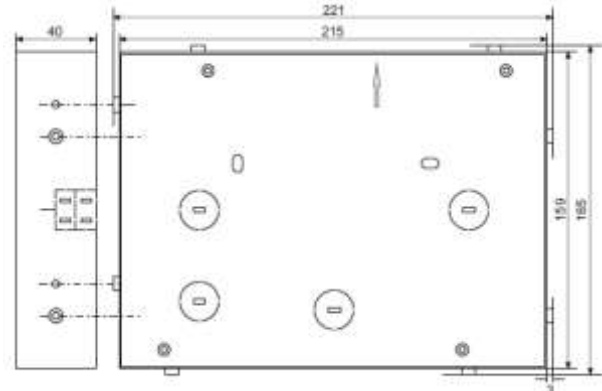
Размеры металлической коробки для монтажа клавиатур на кирпичную стену
