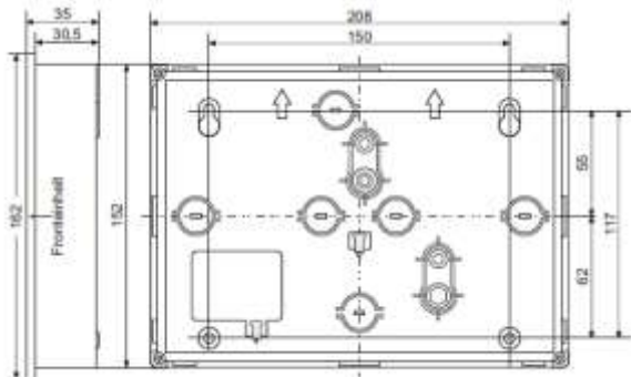
Размеры заднего глубокого кожуха
