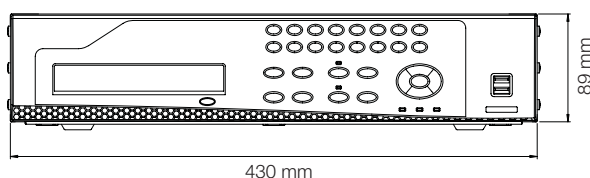
Vista frontale (16 canali)
