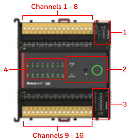
16 Digital Inputs
