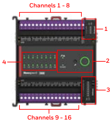
16 Universal I/O
