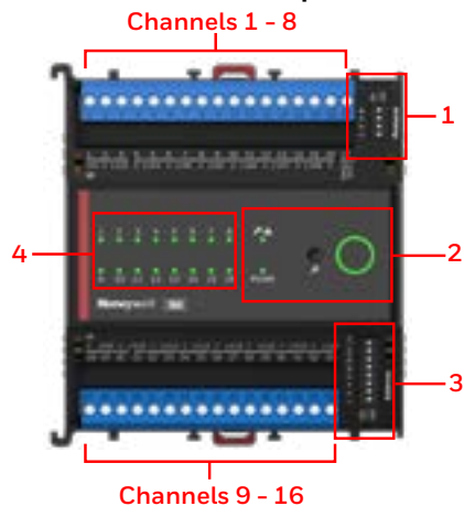
16 Universal Inputs
