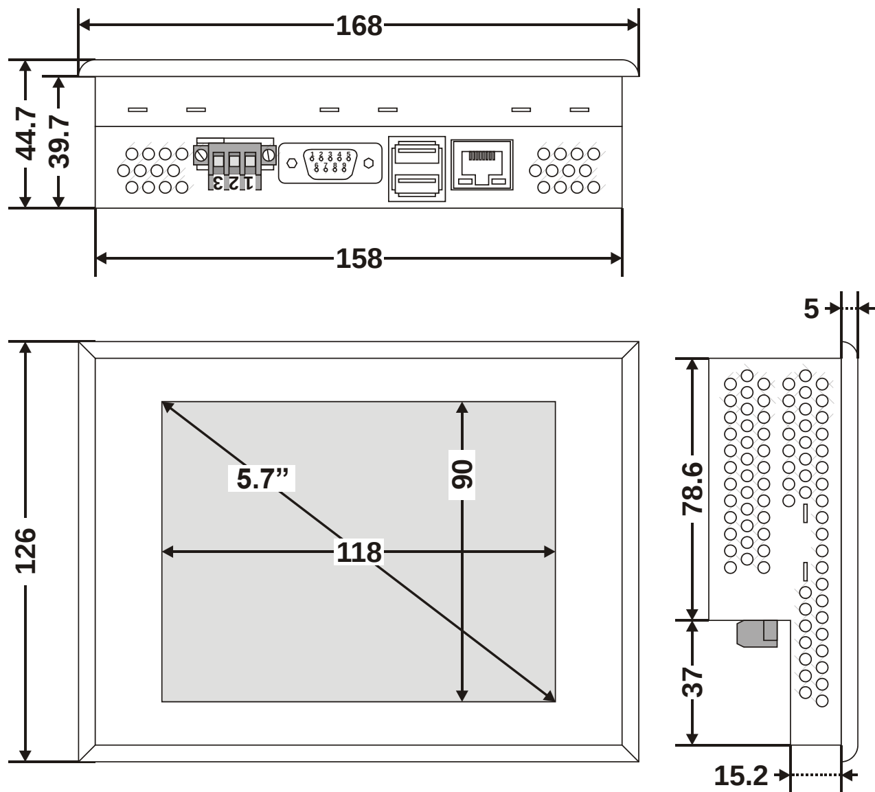
Fig. 3. Excel Touch, dimensiones (en mm)
