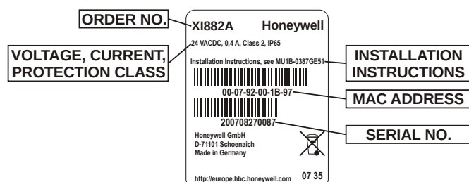
Fig. 2 Placa de fabricación
