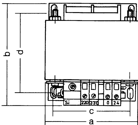
Abb. 2: Abmessungen CRT 6 und CRT 12
