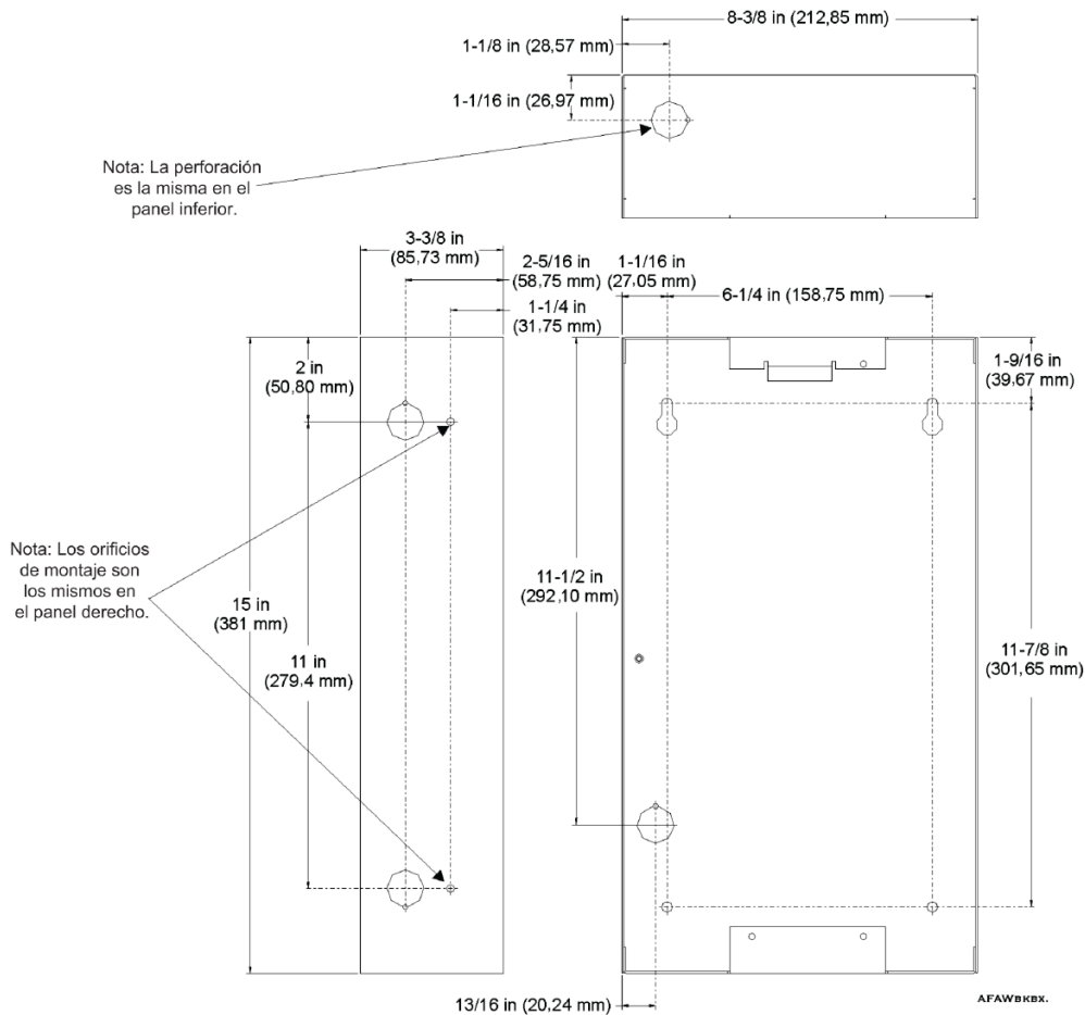
Dimensiones de la caja de montaje
