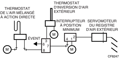
Fig. 7. Fonctionnement type d'une installation avec un RP471 servant à faire passer la commande d'un registre d'air extérieur de la position air mélangé à la position ouverture minimale lorsque la température extérieure dépasse une certaine valeur.
