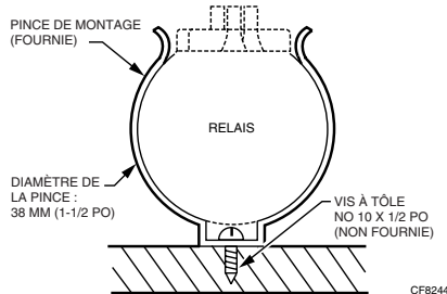
Fig. 2. Montage en surface du RP471A avec une pince de montage.
