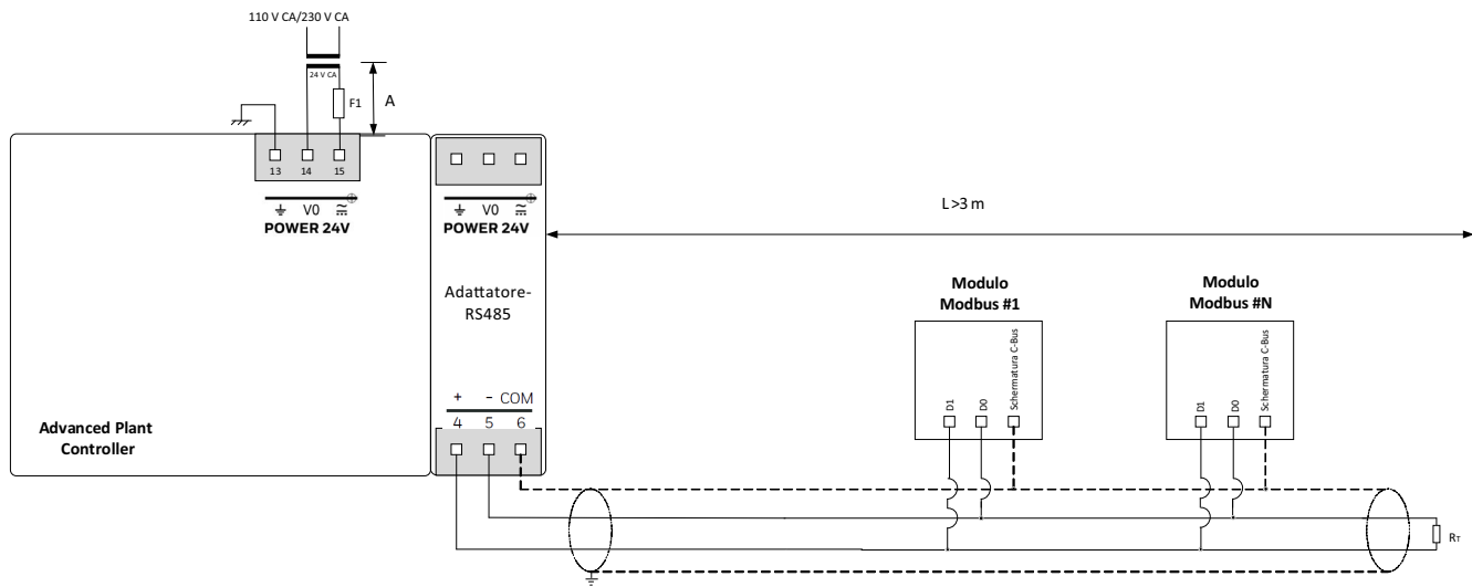
Figura 140. Collegamento ( L > 3 m) di RS485-R a un Modbus
