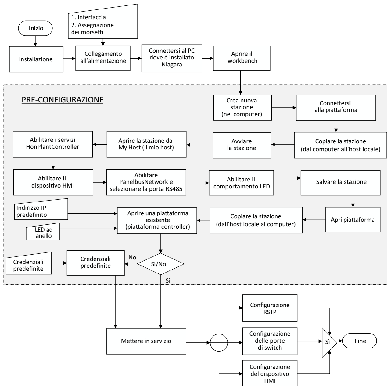
Figura 17. Diagramma del flusso di lavoro 2
