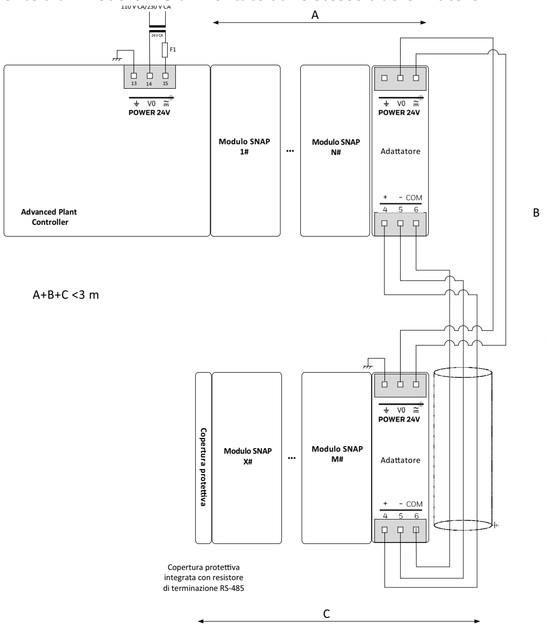
Figura 143. Collegamento (L < 3 m) di RS485-R a un bus - modulo I/O
