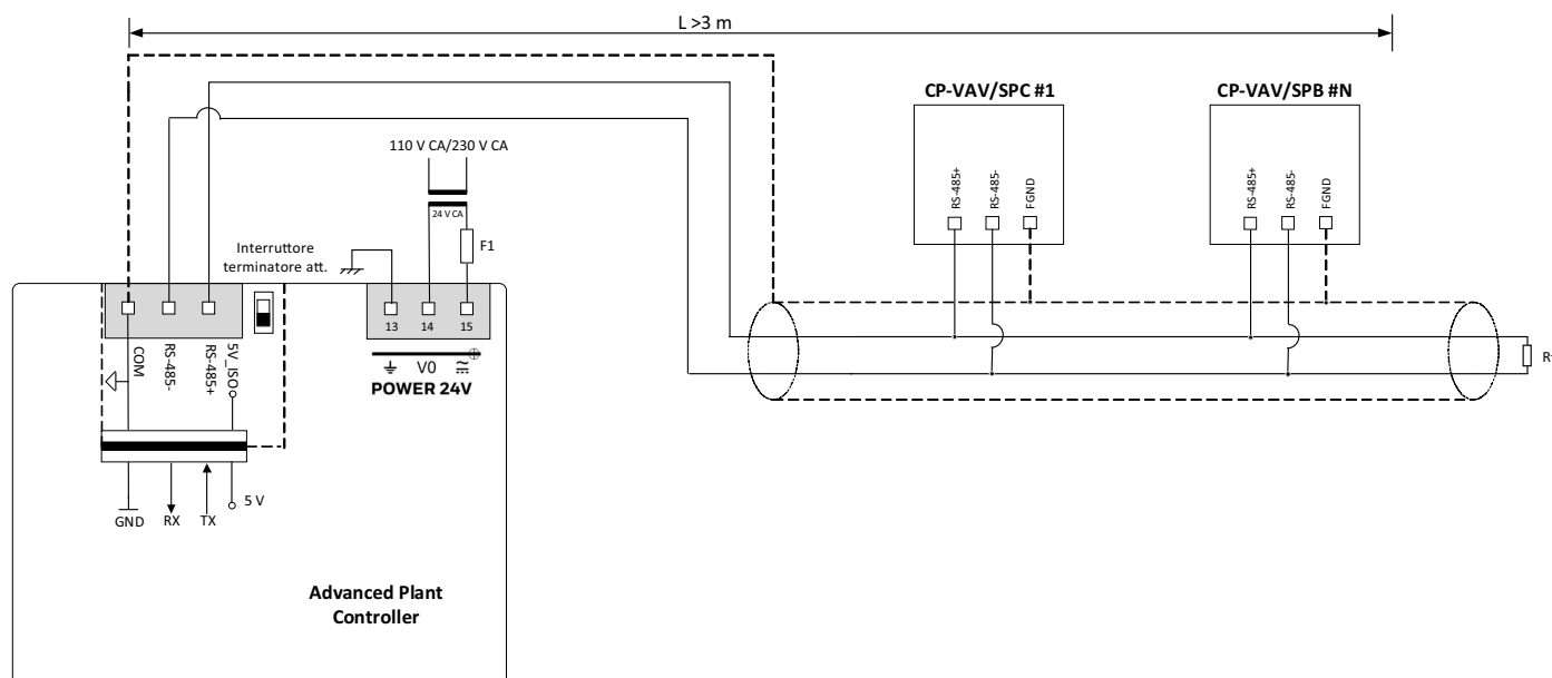
Figura 134. Collegamento ( L > 3 \text{ m} ) delle interfacce RS485 1, 2 o 3 (illustrata l'interfaccia RS485 1) a un bus BACnet
