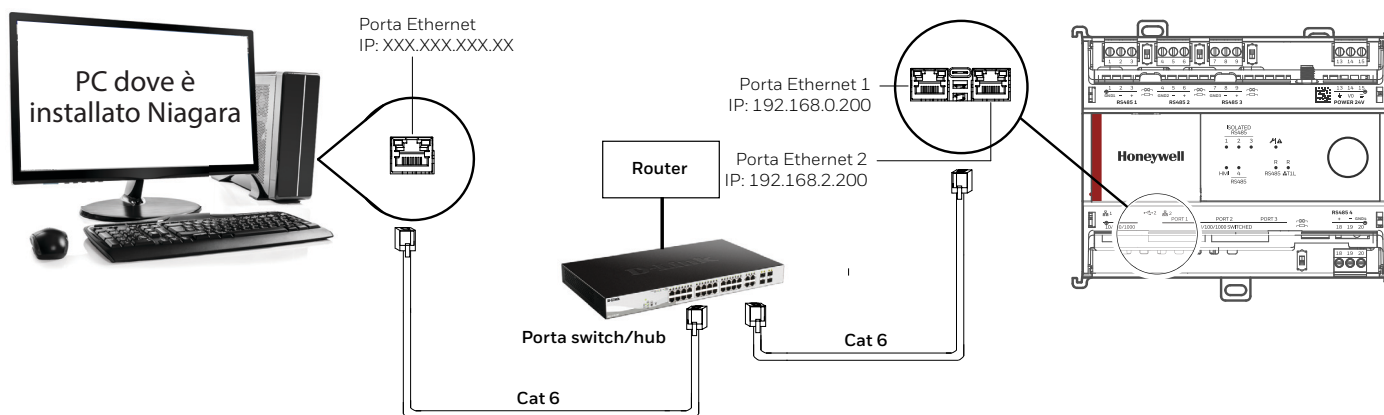
Figura 24. Collegamento tramite hub o switch Ethernet
