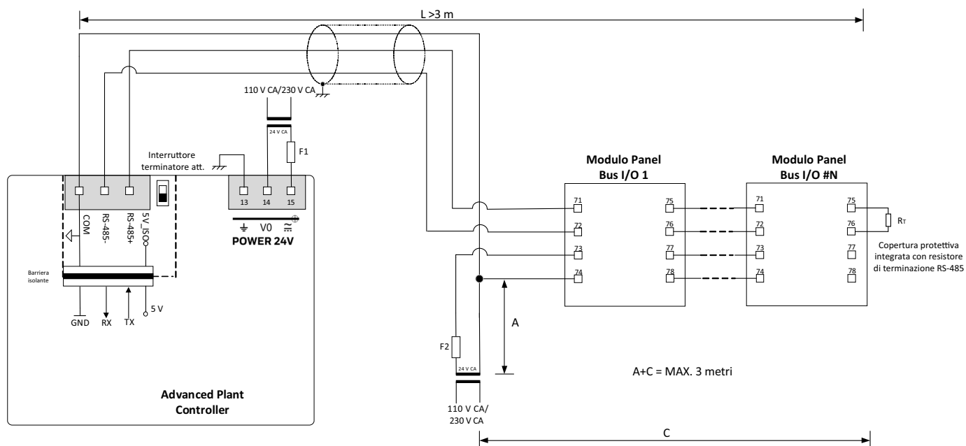
Figura 130. Collegamento ( L > 3 m) delle interfacce RS485 1, 2 o 3 (illustrata l'interfaccia RS485 1) a un Panel Bus
