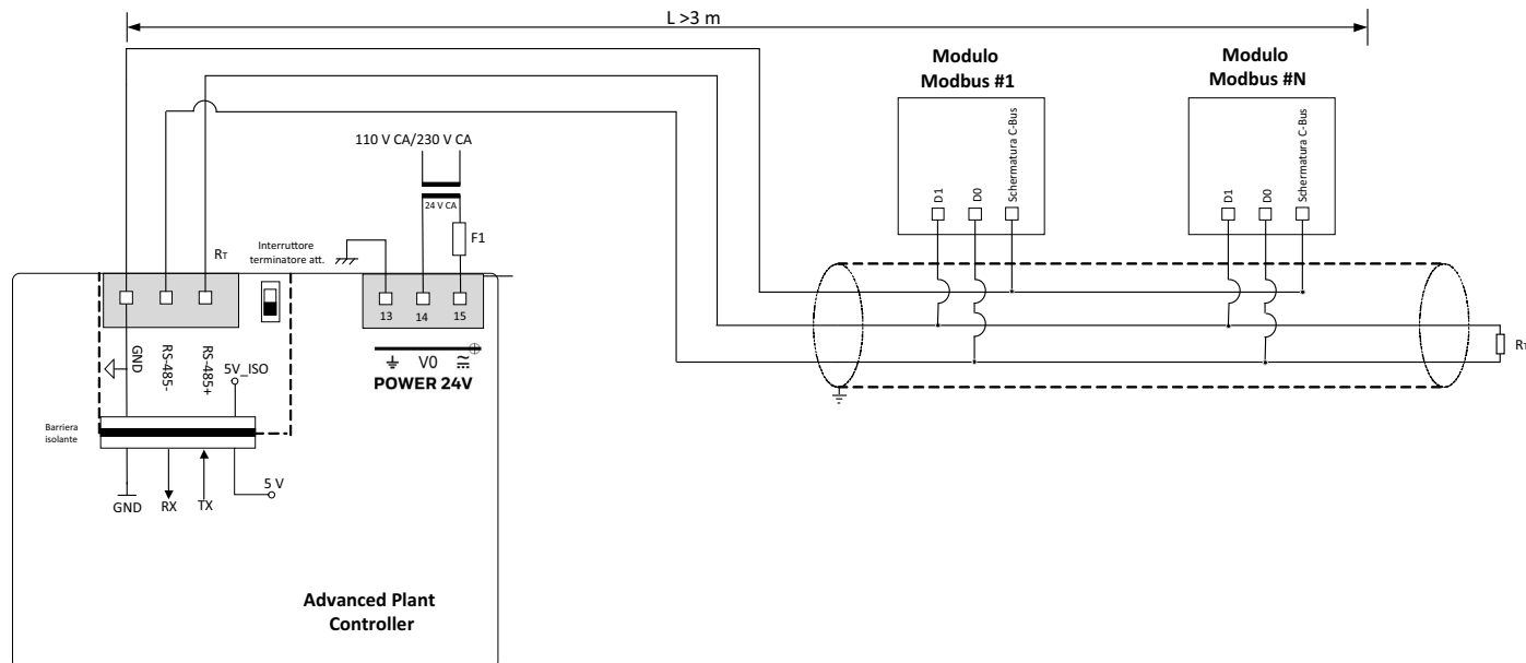
Figura 139. Collegamento ( L > 3\text{ m} ) delle interfacce RS485 1, 2 o 3 (illustrata l'interfaccia RS485 1) a un Modbus
