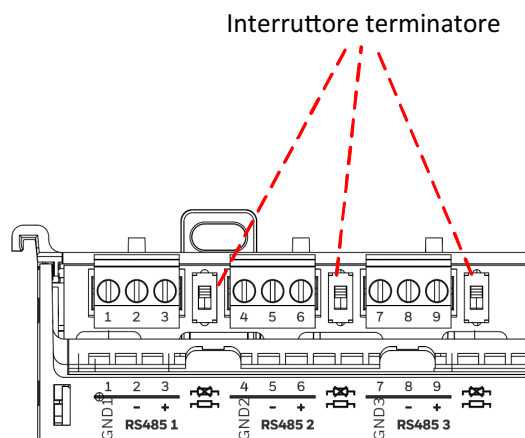
Figura 10. Interruttore terminatore
