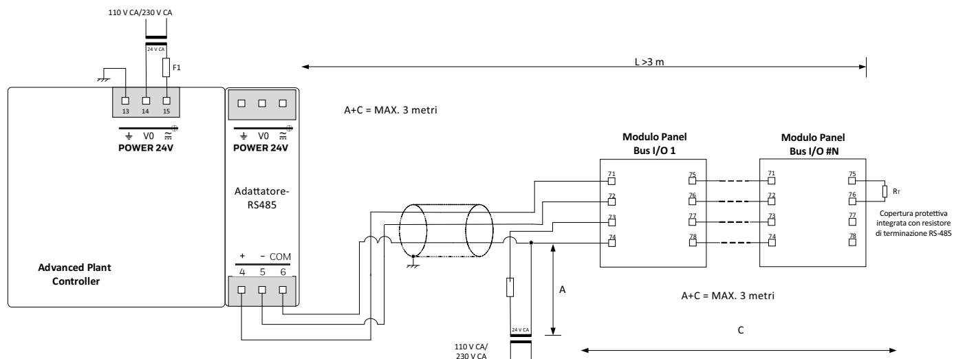
Figura 131. Collegamento ( L > 3 \text{ m} ) dell'interfaccia RS485 R a un Panel Bus
