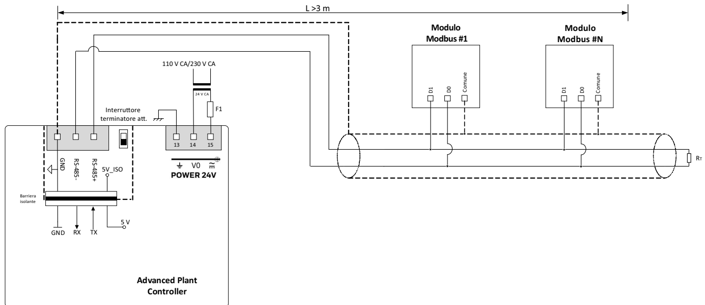
Figura 138. Collegamento ( L > 3 m) delle interfacce RS485 1, 2 o 3 (illustrata l'interfaccia RS485 1) a un Modbus
