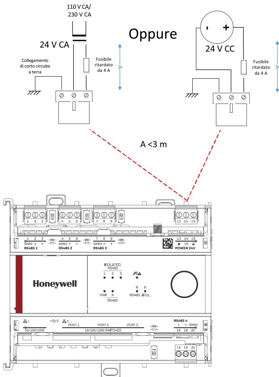
Figura 7. Collegamento all'alimentazione e a terra
