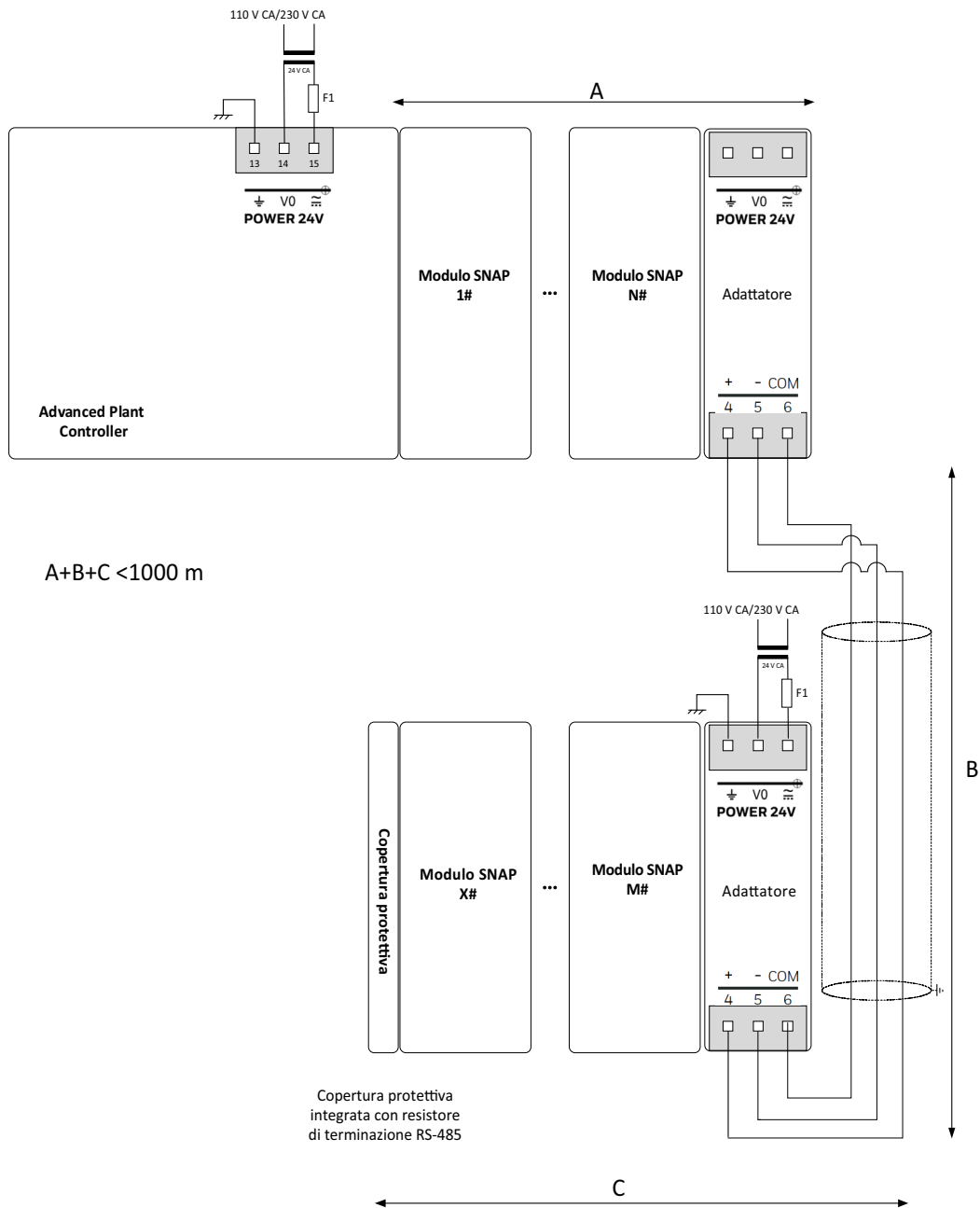
Figura 142. Collegamento ( L > 3 m) di RS485-R a un bus I/O - modulo I/O
