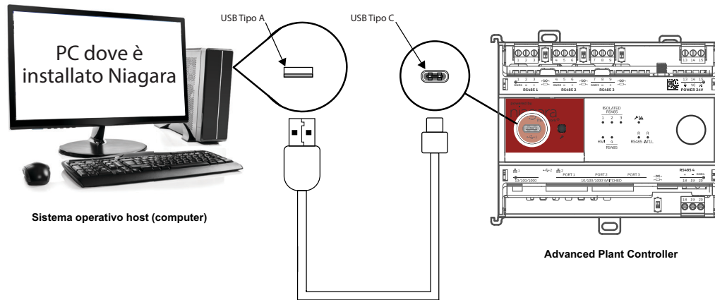
Figura 19. Collegamento USB dal computer al controller
