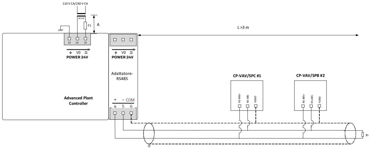
Figura 136. Collegamento ( L > 3 m) di RS485-R a un bus BACnet
