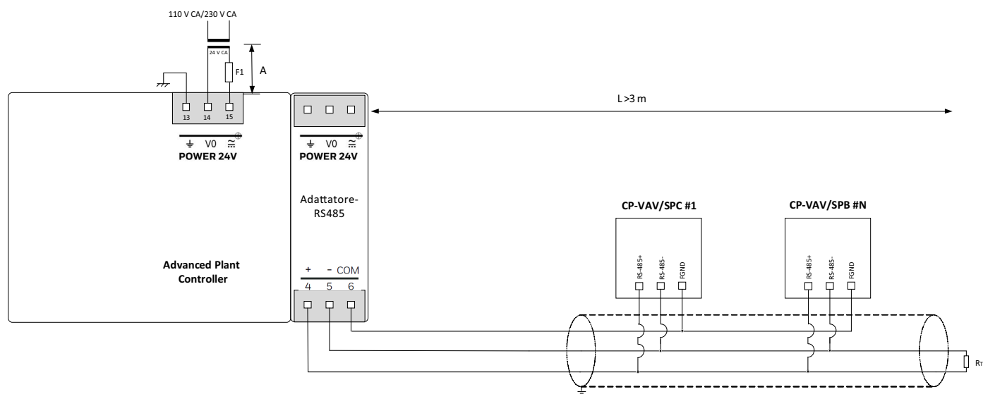
Figura 137. Collegamento ( L > 3 m) di RS485-R a un bus BACnet
