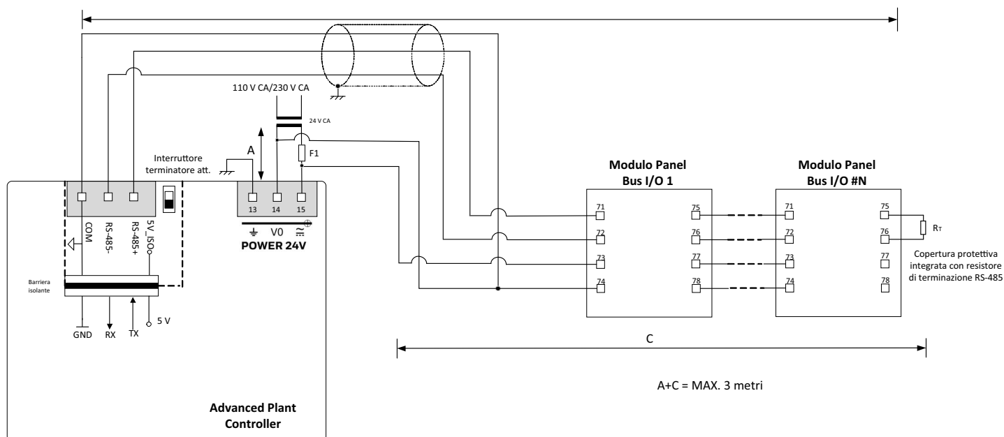
Figura 132. Collegamento ( L < 3 m) delle interfacce RS485 1, 2 o 3 (illustrata l'interfaccia RS485 1) a un Panel Bus
