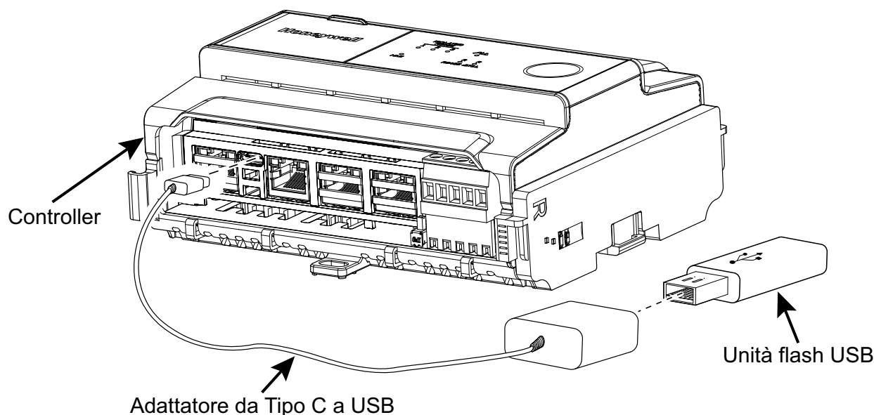
Figura 123. Collegamento della porta USB all'unità flash USB
