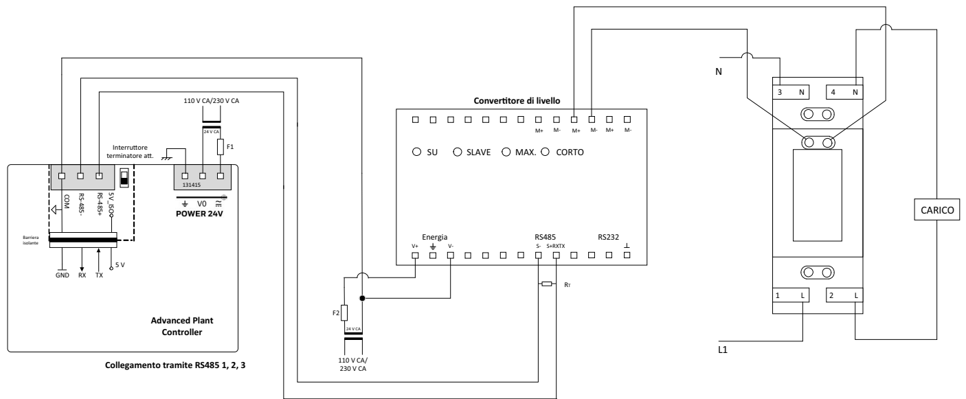
Figura 144. Collegamento a M-Bus tramite convertitore di livello
