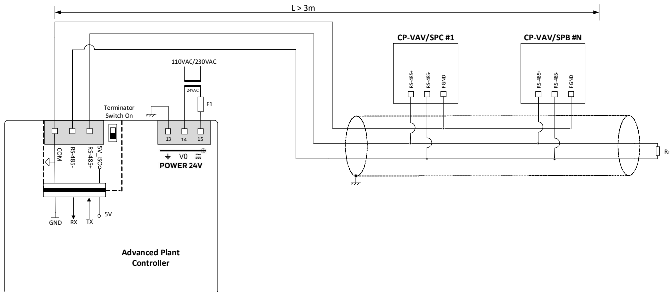
Figura 135. Collegamento ( L > 3\text{ m} ) delle interfacce RS485 1, 2 o 3 (illustrata l'interfaccia RS485 1) a un bus BACnet
