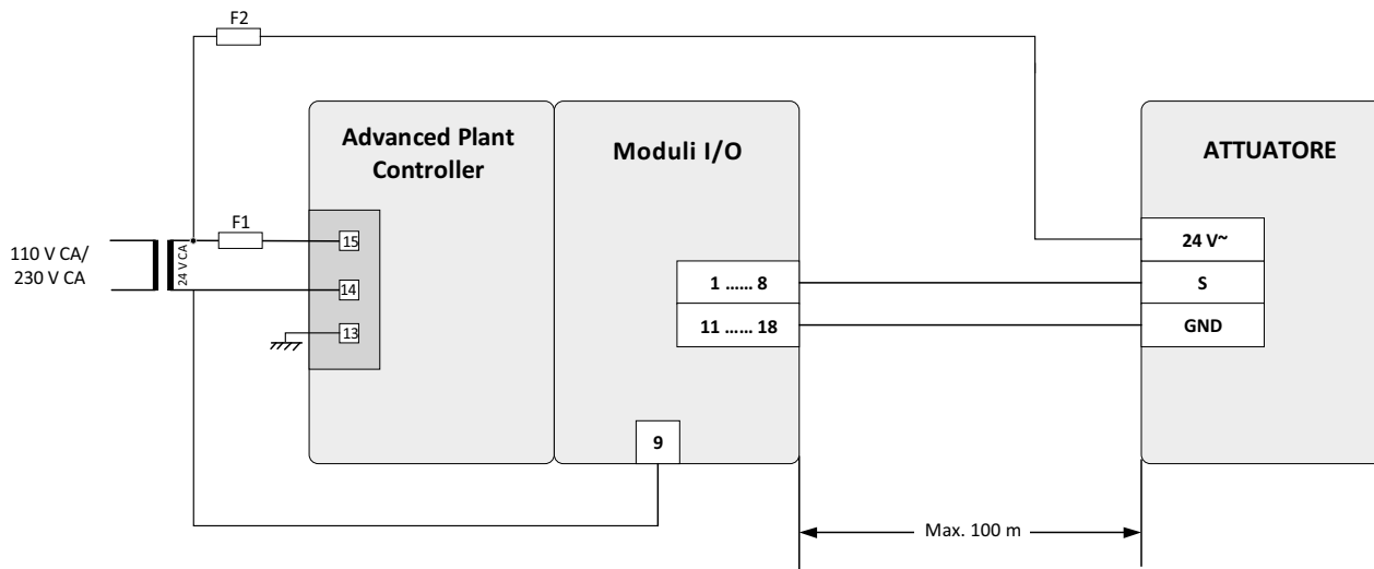
Figura 5. Alimentazione di dispositivi di campo tramite modulo I/O Panel Bus
