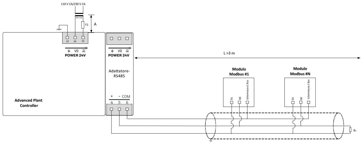
Figura 141. Collegamento ( L > 3 m) di RS485-R a un Modbus
