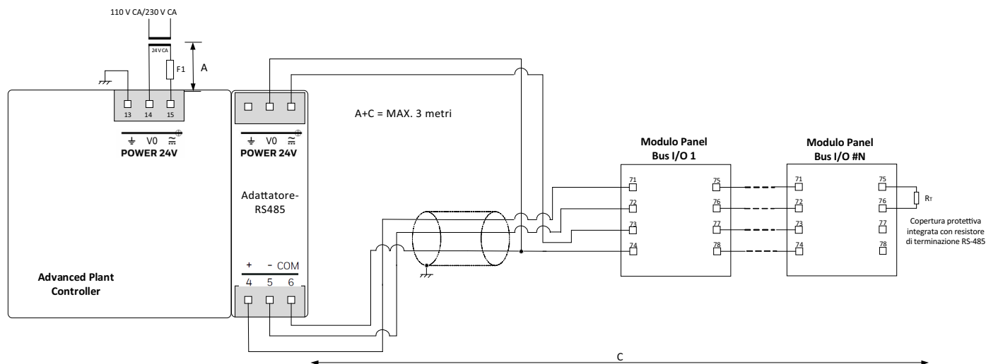
Figura 133. Collegamento ( A + C < 3 \text{ m} ) dell'interfaccia RS485 R a un Panel Bus
