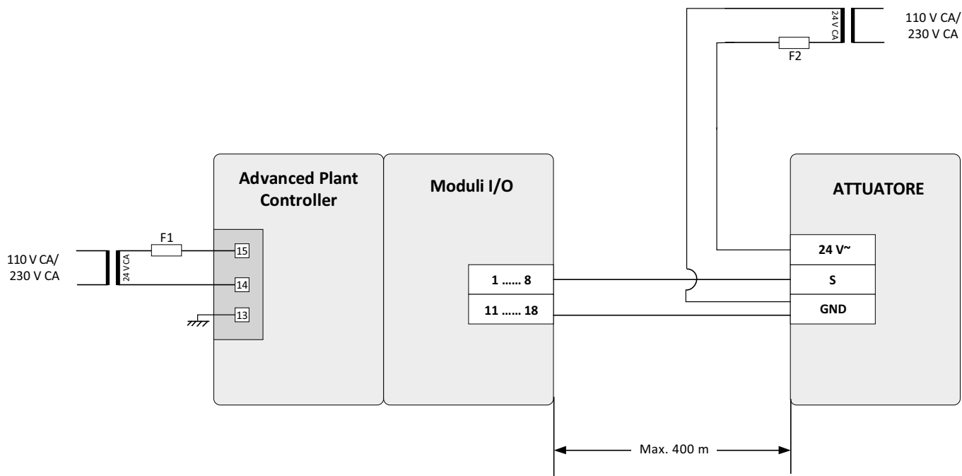
Figura 6. Alimentazione di dispositivi di campo mediante trasformatore separato
