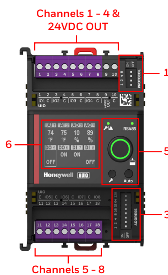
8 UIO - HOA
