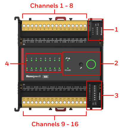
16 Digital Inputs
