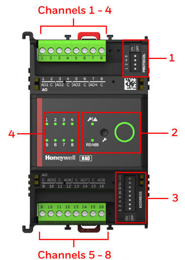
8 AO
