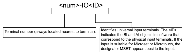
Fig. 15 UIO terminals
