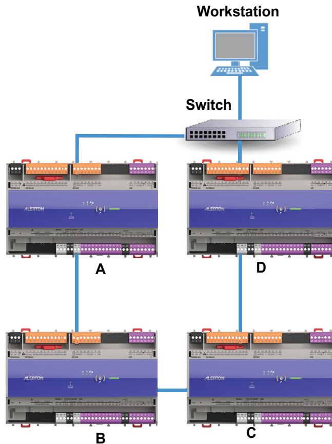
Fig. 59 RSTP Scenario
