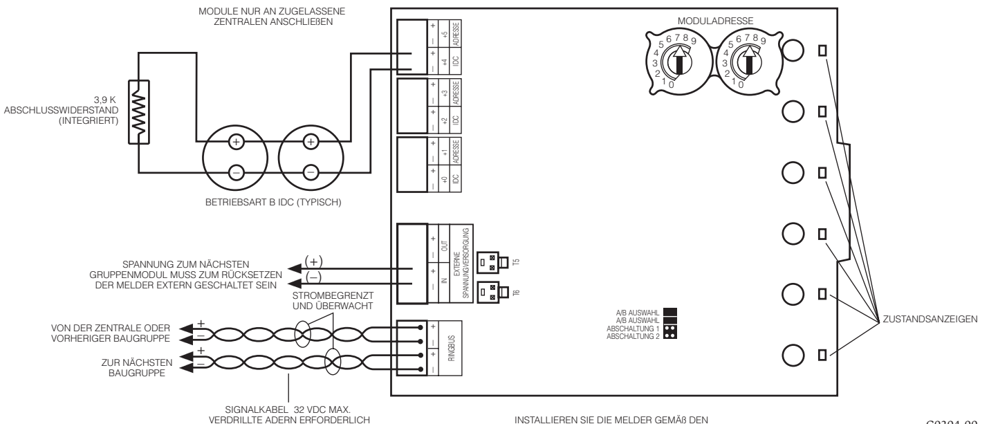
ABBILDUNG 1. UM EINE GEMEINSAME SPANNUNGSVERSORGUNG FÜR MEHRERE CZ-6 MODULE EINZUSETZEN, SCHLIESSEN SIE DAS STECKKABEL ZUR SPANNUNGSVERSORGUNG VON T5 ODER T6 AN T5 ODER T6 DES BENACHBARTEN CZ-6 MODULES AN
