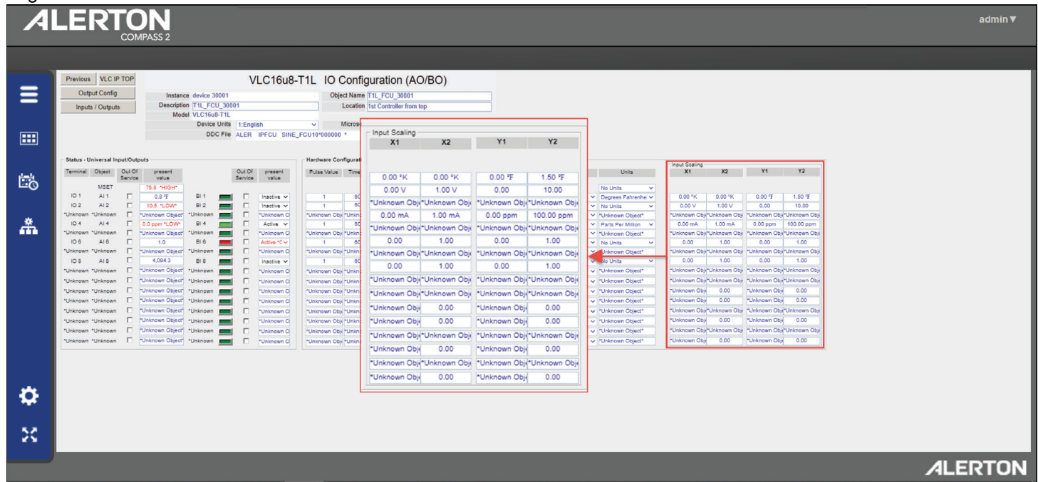
Fig. 63 Input scaling
