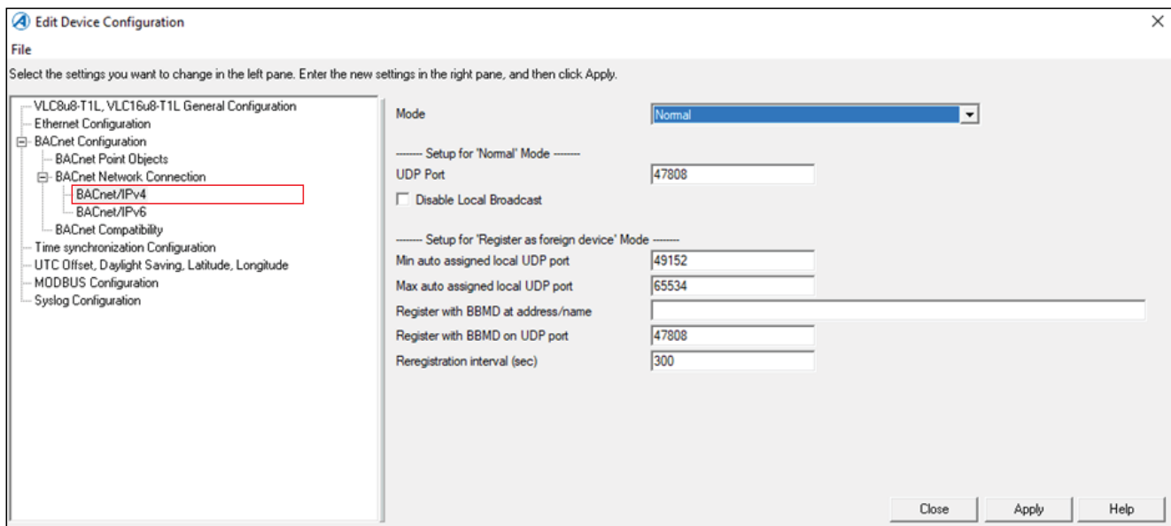
Fig. 34 BACnet/IPv4
