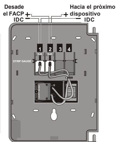
Alambrado de la NBG-12, 12L, 12LSP de Acción Doble
