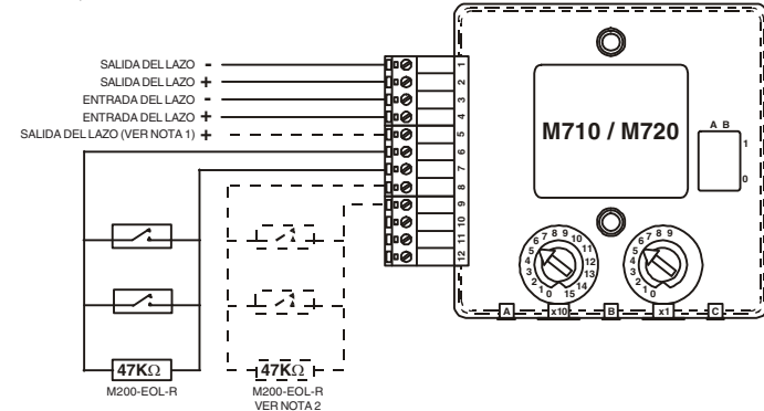
FIGURE 3: CONEXIONES DE LOS MÓDULOS M710 DE ENTRADA ÚNICA Y M720 DE ENTRADA DOBLE
