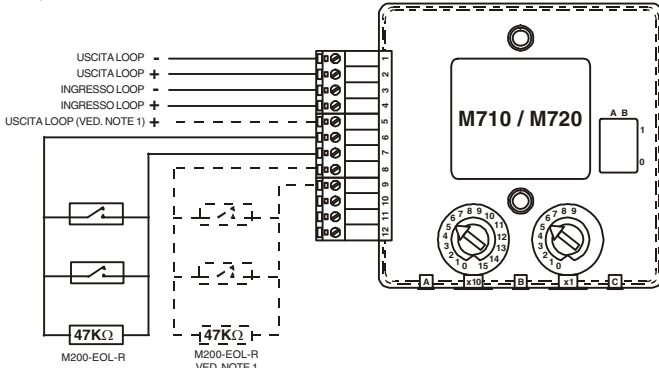
FIGURA 3: CABLAGGIO DEL MODULO A INGRESSO SINGOLO M710 E A INGRESSO DOPPIO M720
