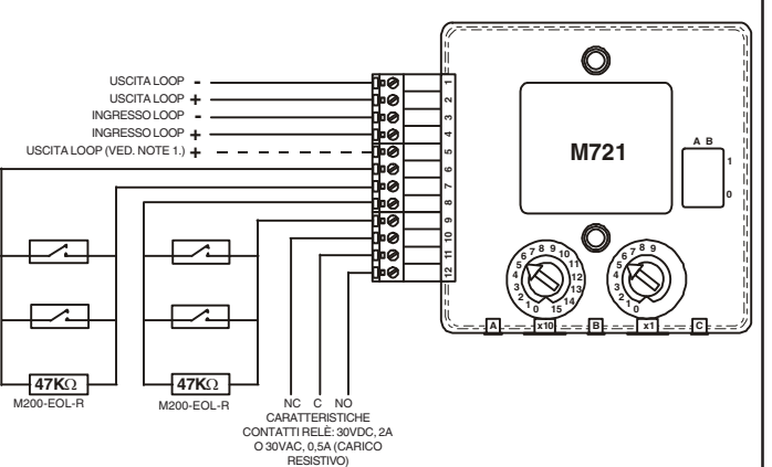
FIGURA 4: CABLAGGIO DEL MODULO A USCITA SINGOLA E DOPPIO INGRESSO M721
