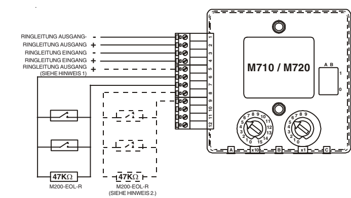
ABBILDUNG 3: ANSCHLUSS DES ÜBERWACHUNGSMODULES M710 UND M720
