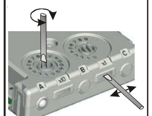
FIGURA 2: SWITCH ROTATIVI PER INDIRIZZAMENTO DECIMALE
