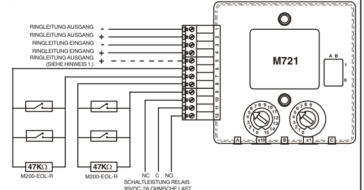
ABBILDUNG 4: VERDRAHTUNG DES M721 ÜBERWACHUNGSMODUL MIT 2 EINGÄNGEN UND EINEM AUSGANG
