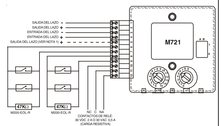
FIGURA 4: CONEXIONES DEL MÓDULO DE ENTRADA DOBLE Y SALIDA ÚNICA M721
