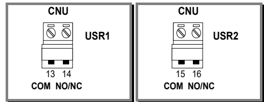
Salidas USR1 - USR2
