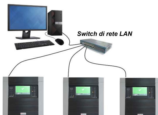
Sistema con più centrali
