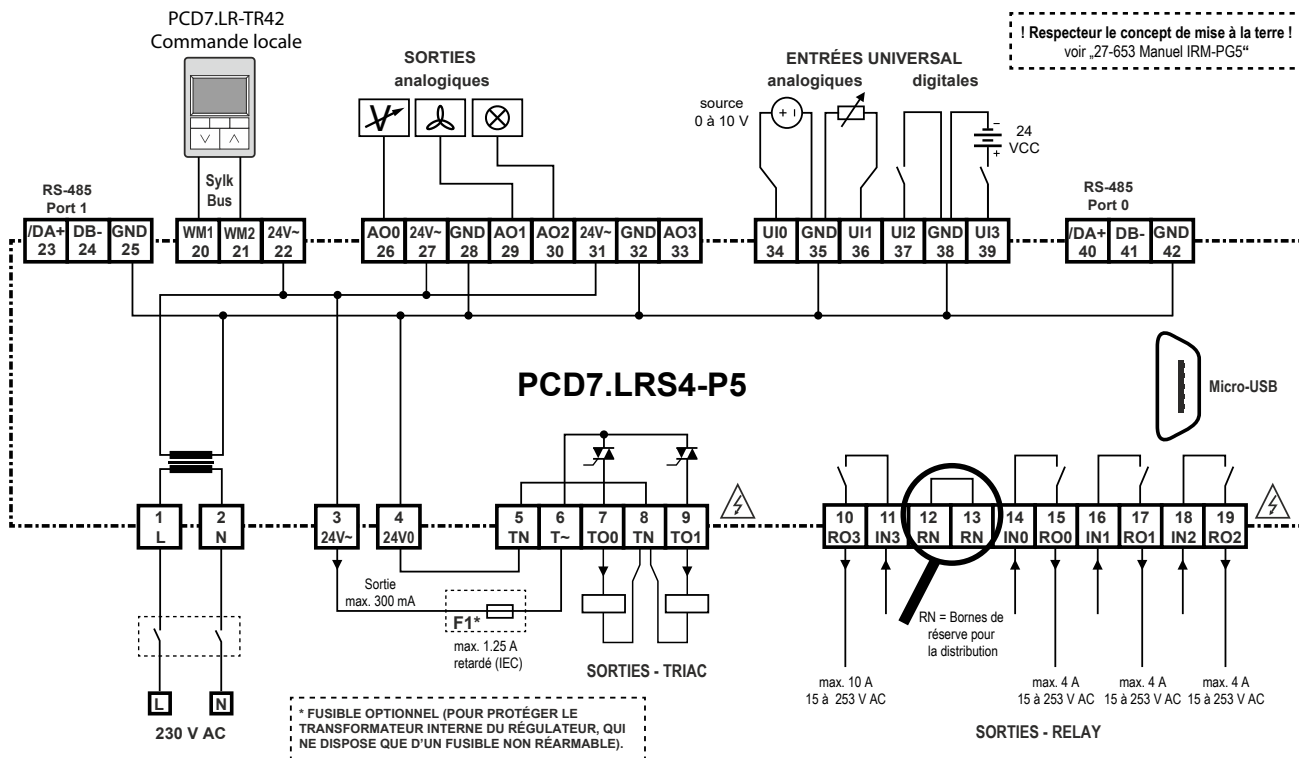
Exemple de câblage PCD7.LRS4-P5
