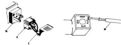
Abb. 2. Verdrahtung
