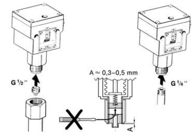
Abb. 3. Druckanschluß
