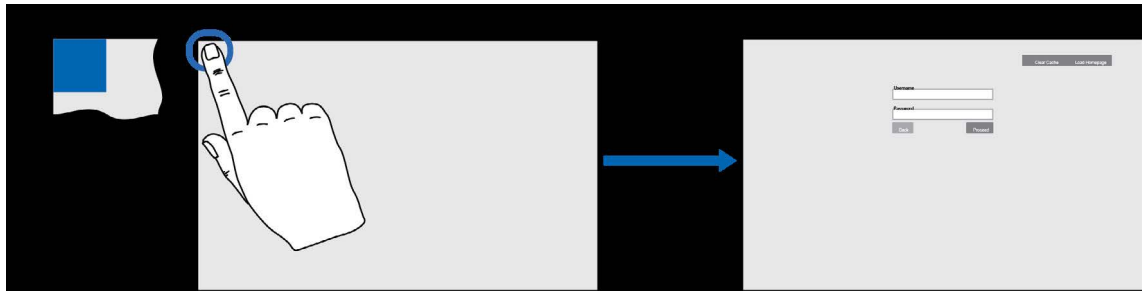
Fig. 7 Login screen
