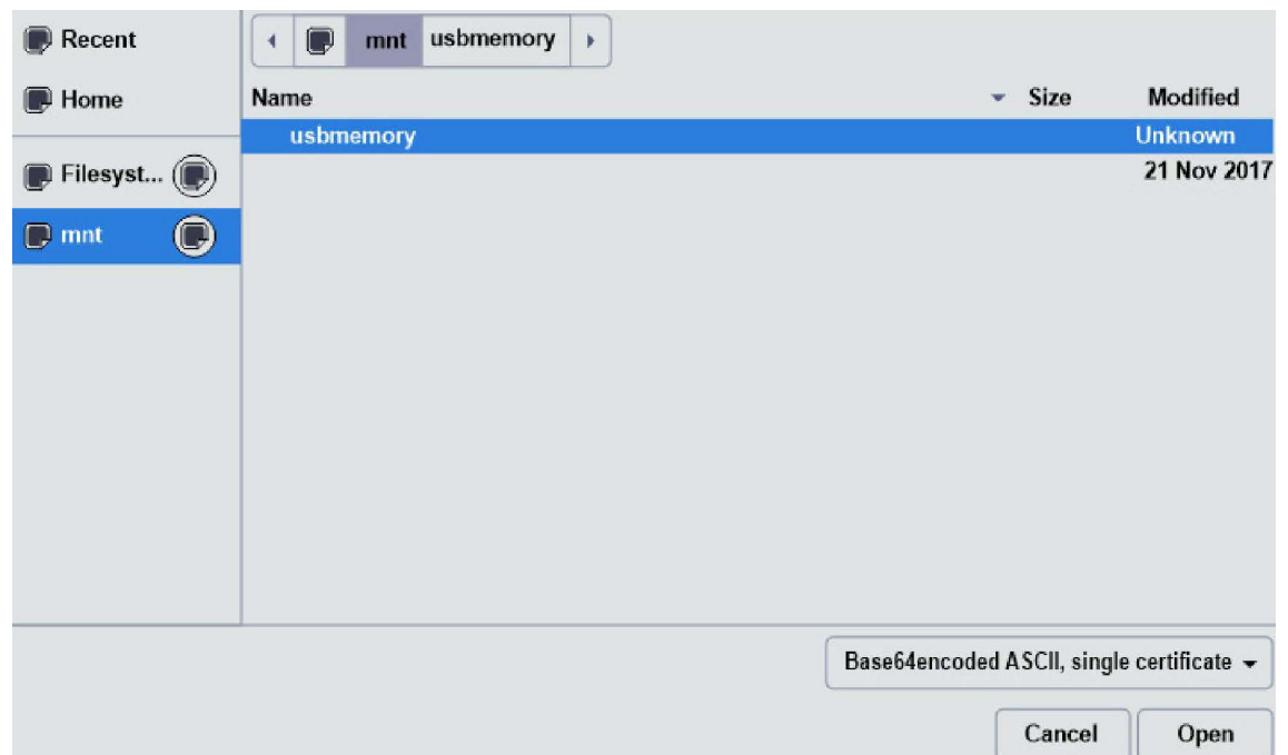
Fig. 47 mnt
