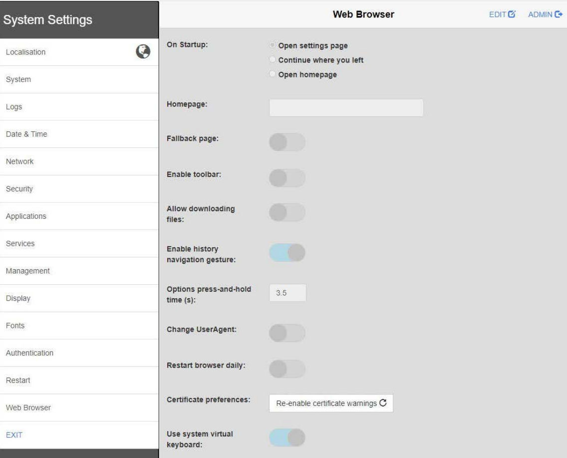
Fig. 27 Web Browser
