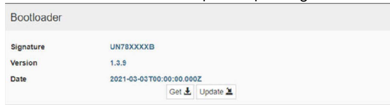
Fig. 28 Bootloader
