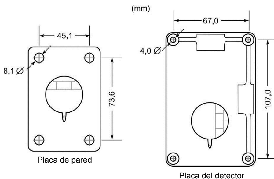
Figura 17. Dimensiones de la placa de conexiones del kit de montaje giratorio SM21
