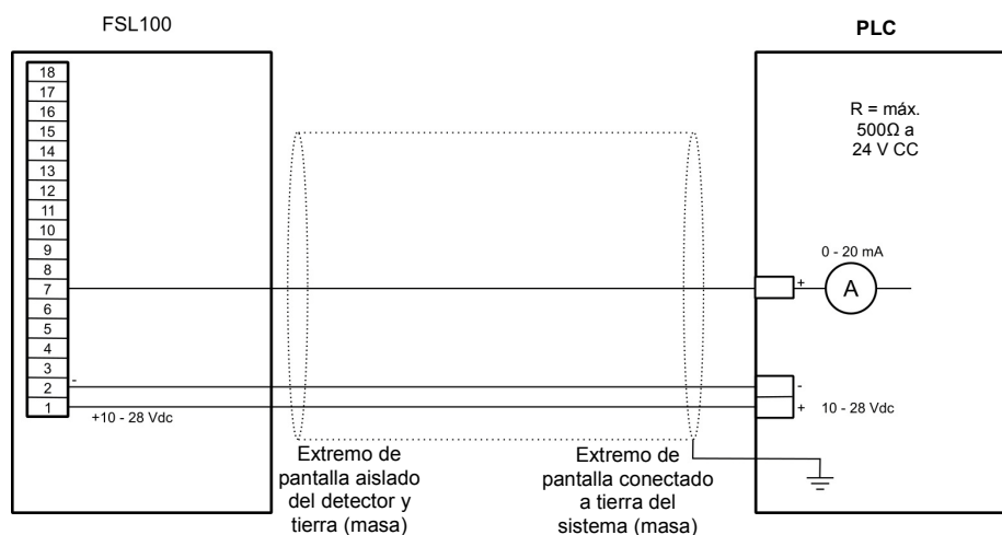
Figura 12. Cableado a un PLC
