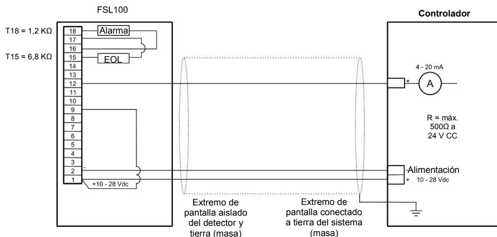
Figura 13. Cableado a una salida de corriente no aislada (fuente) de 4 a 20 mA
