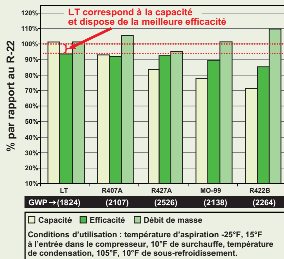
Figure 1. Genetron Performax LT surpasse ses concurrents pour les nouvelles installations de supermarché et les mises à niveau
