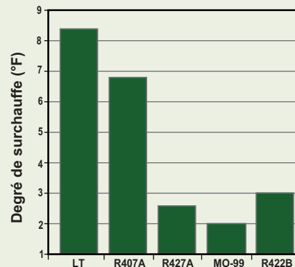
Figure 2. Dans une analyse de remplacement direct, Genetron Performax LT a préservé la surchauffe, protégé les compresseurs et assuré l'utilisation optimale de la capacité de réfrigération.
