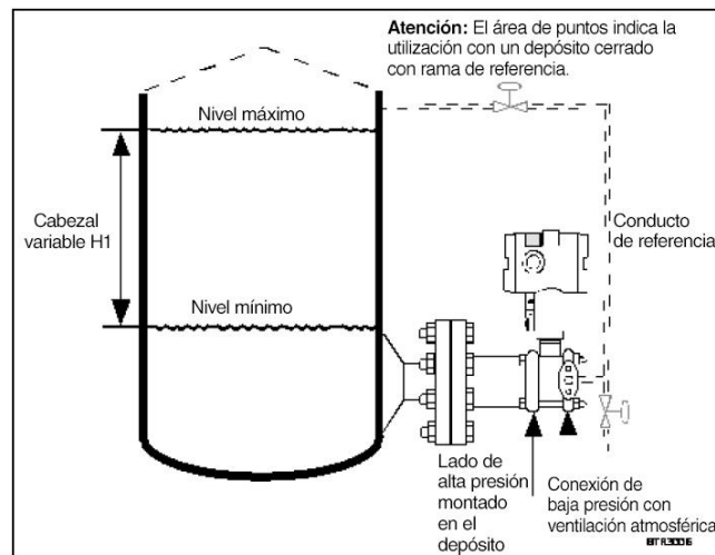
Figura 3: Montaje típico de un transmisor de nivel montado en brida
