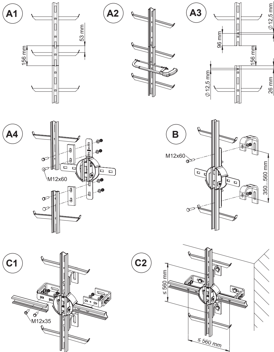
Fig. 2.12 - Table tournante avec 4 supports
