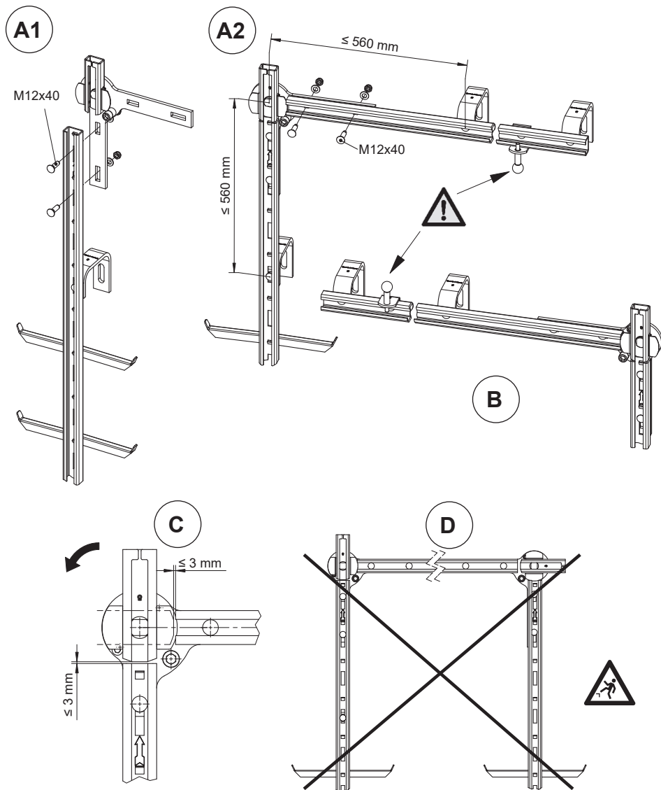
Fig. 2.15 - Table tournante Ho-Ver : A1/ A2: Assemblage et dimensions, version vers la droite - butée vers le bas B: Version vers la gauche - butée vers le haut C: Fonctionnement et écarts D: Assemblage interdit
