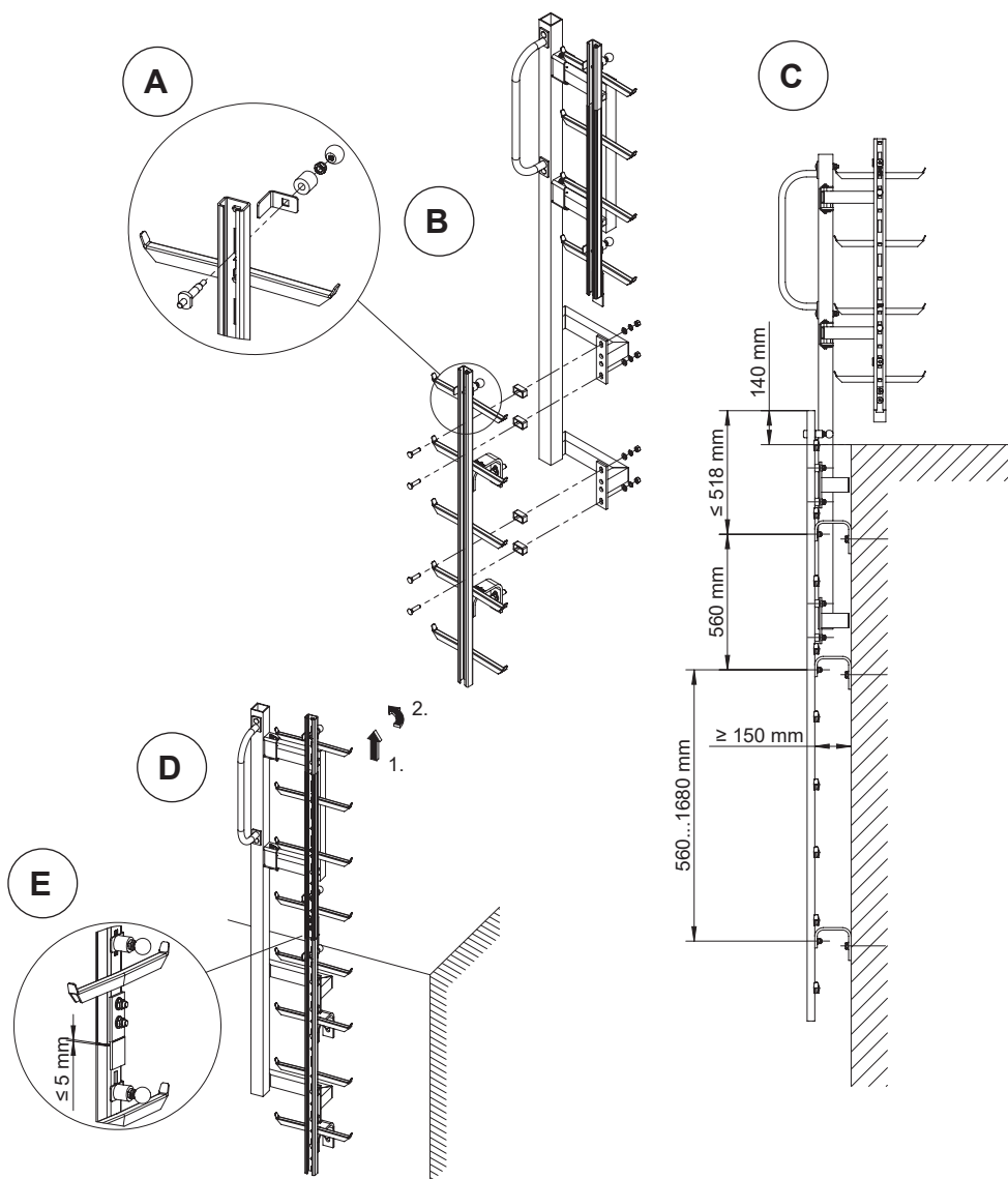
Fig. 2.11 - Sortie de toit :
