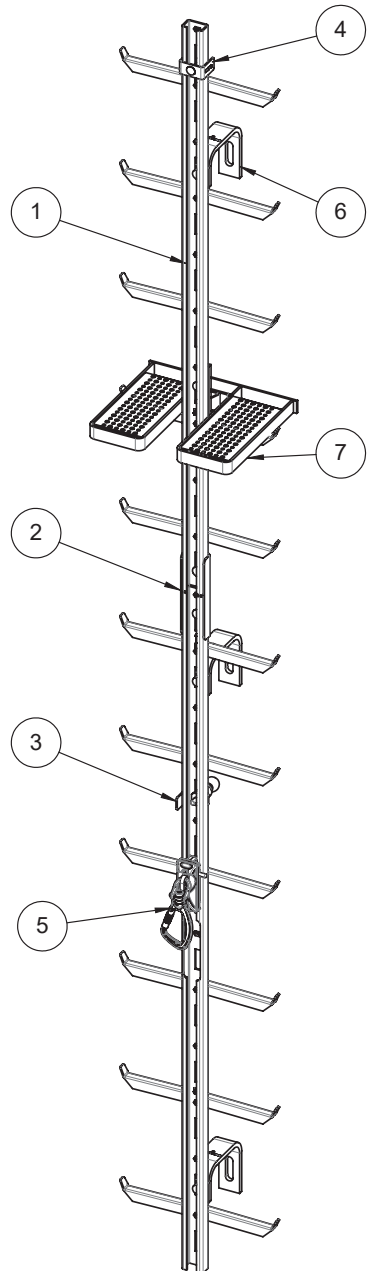
Fig 1.1: Composants typiques du système antichute Söll GlideLoc
