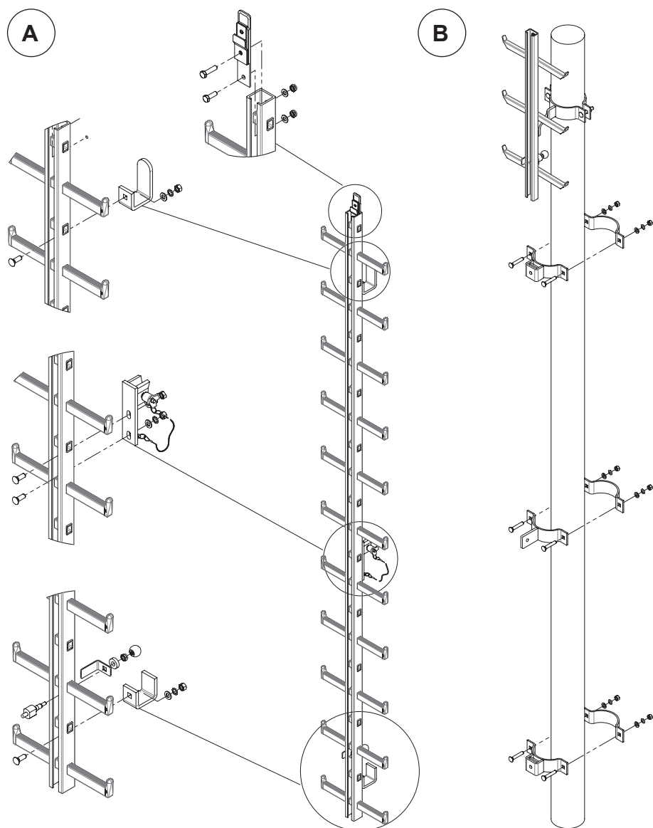
Fig. 2.17 - Échelle d'insertion de l'assemblage A: Supports d'assemblage B: Colliers d'assemblage
