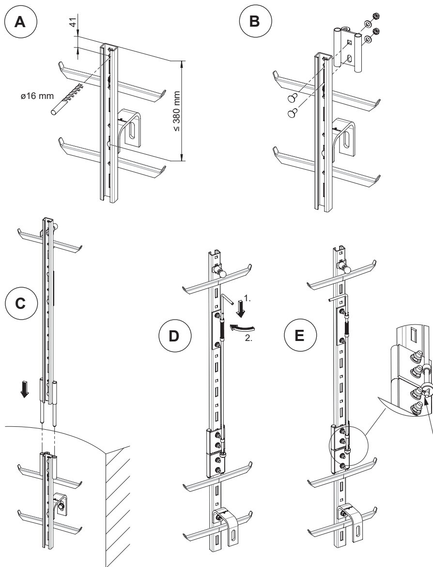
Fig. 2.16 - Dispositif d'entrée d'arbre de l'assemblage :
