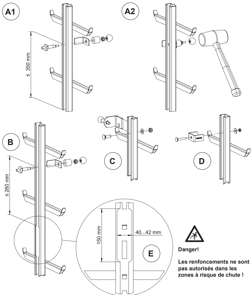
Fig. 2.2 - Installation des butées
