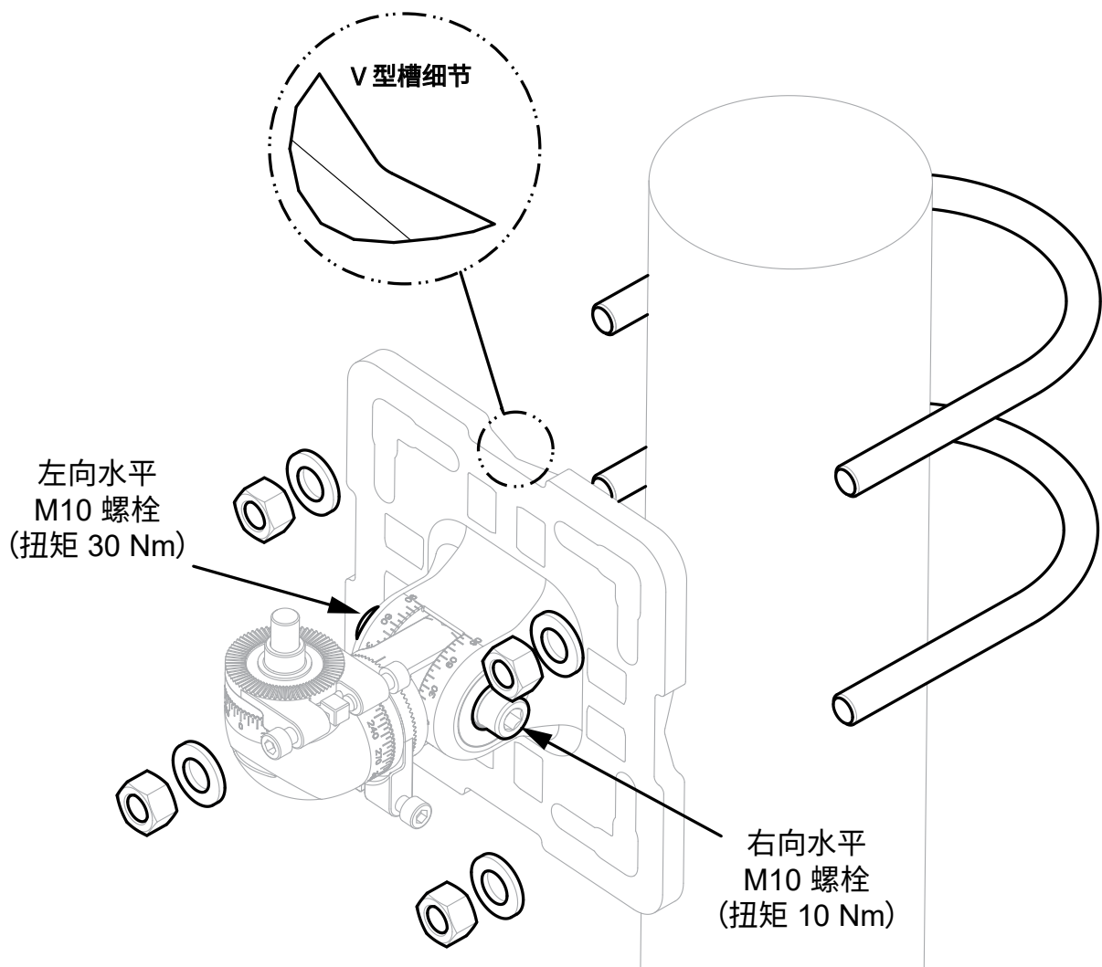
图 10. 使用 U 型螺栓将通用安装支架安装到杆上
