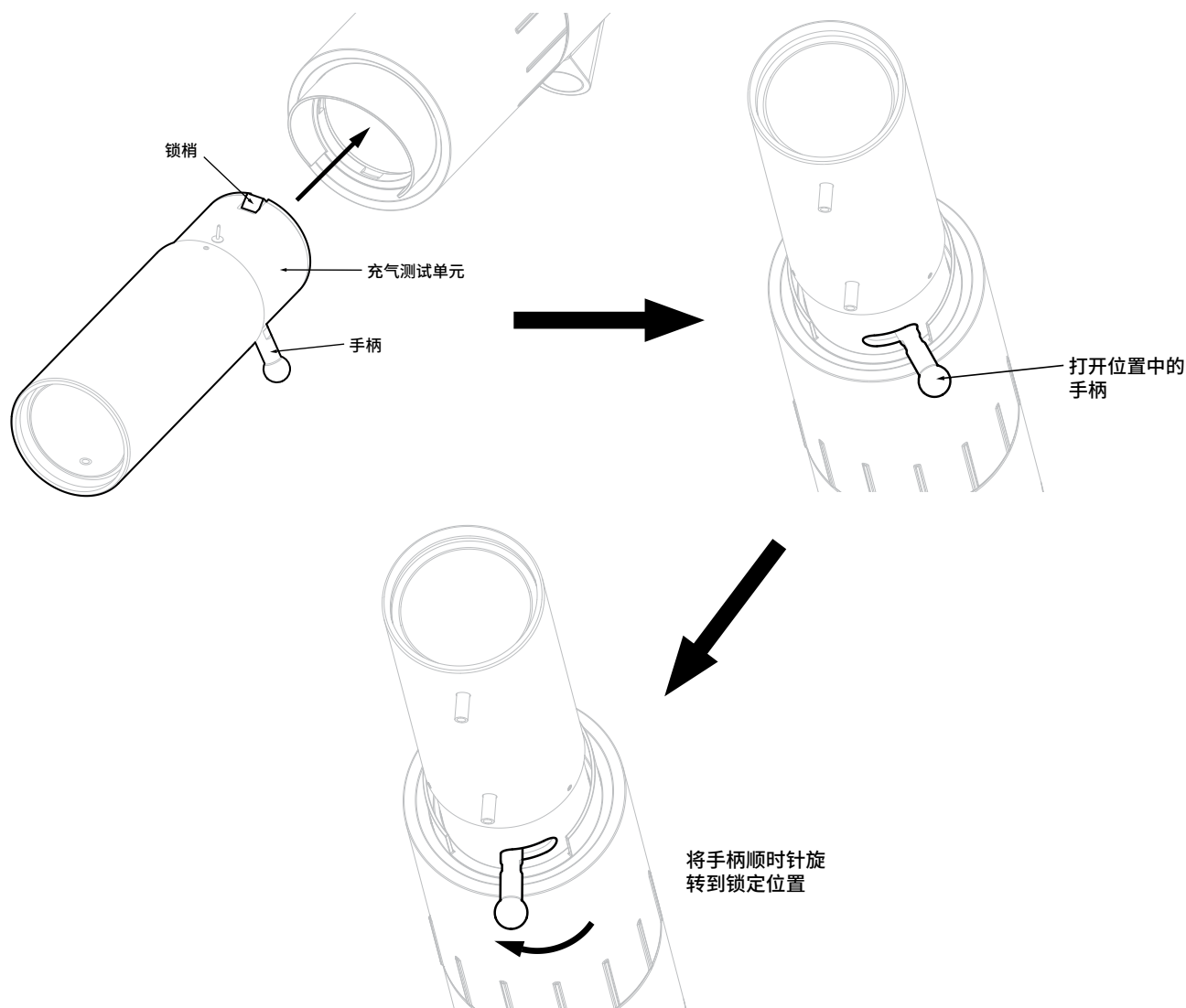
图 39. Connecting 将充气测试单元连接到接收器
