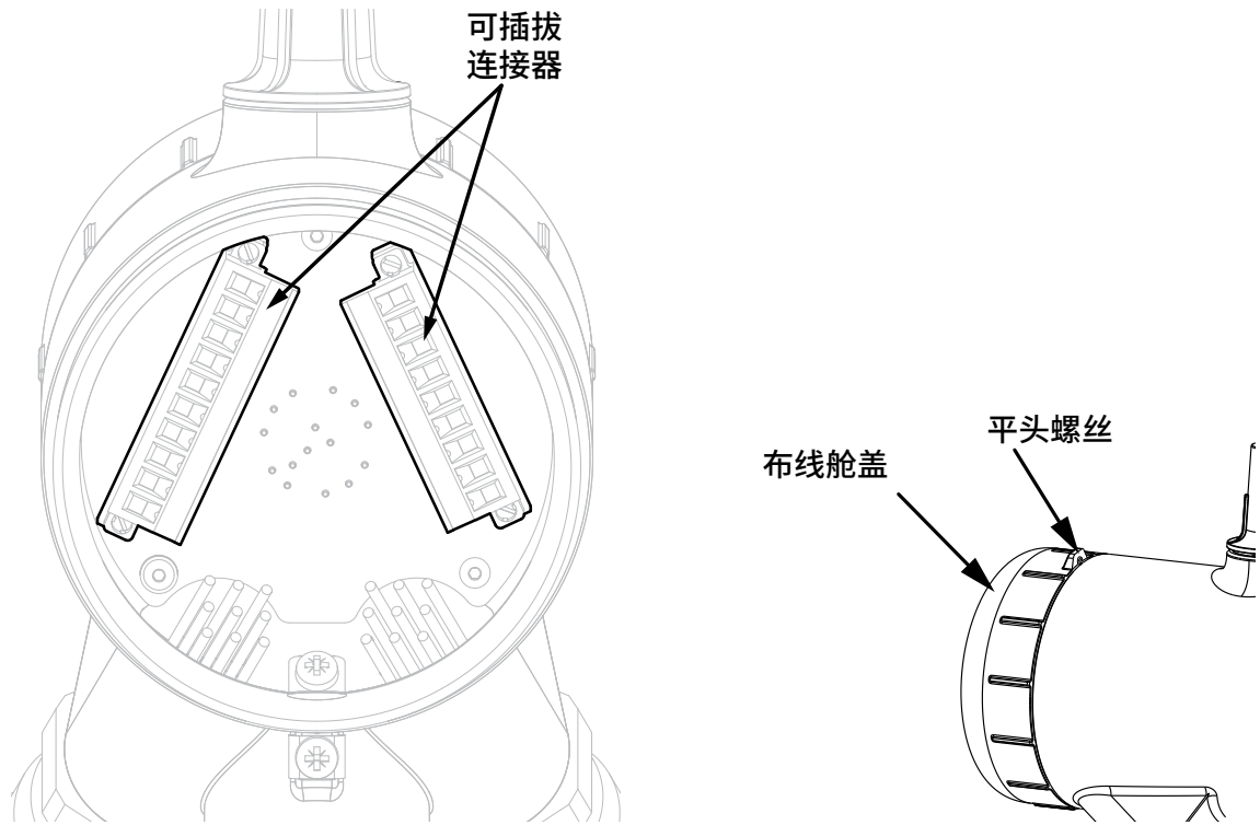
图 16. PCB 端子
