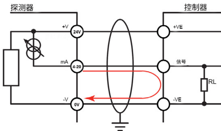
图 27. mA 回路配置作为电流阱
