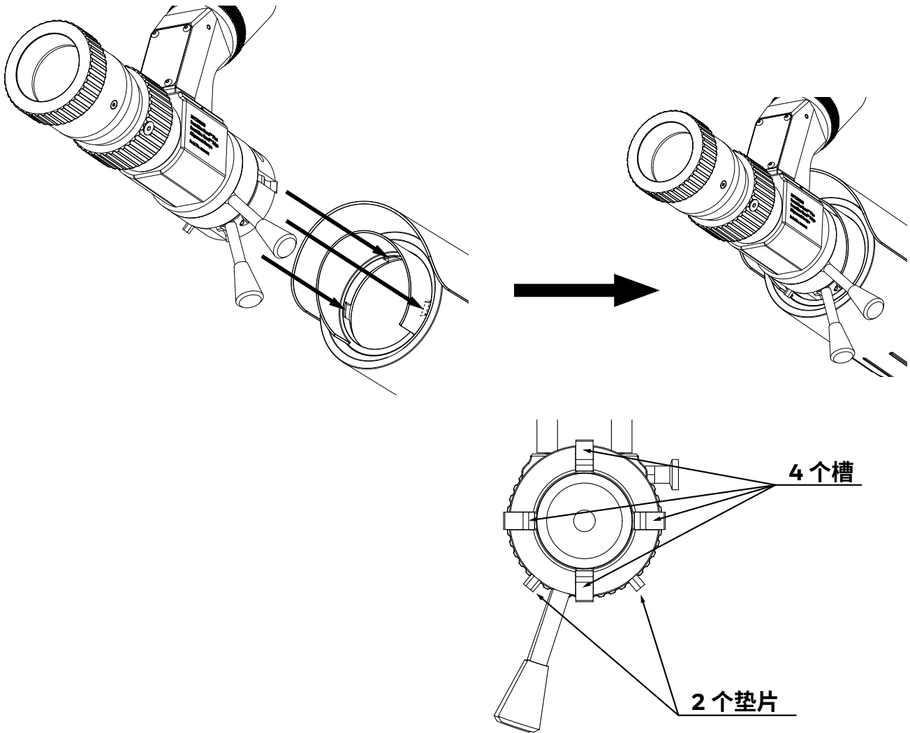
图 32. 将 Alignment Scope 安装到仪器上
