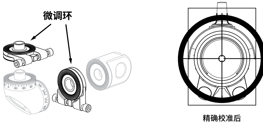
图 36. 微调环和精确校准后的视图
