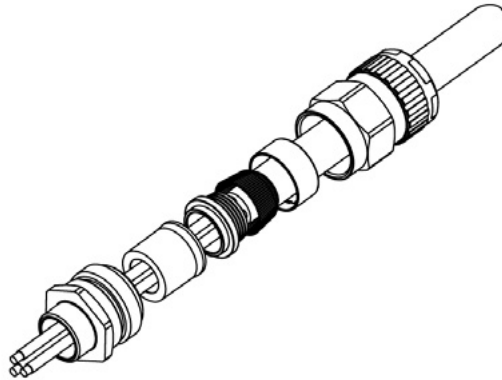
图 13. 电缆密封接头示例
