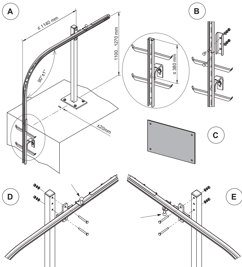
Fig. 2.10 - Zahnutá výměnná kolej: A: Rozměry (výstup vpravo)
