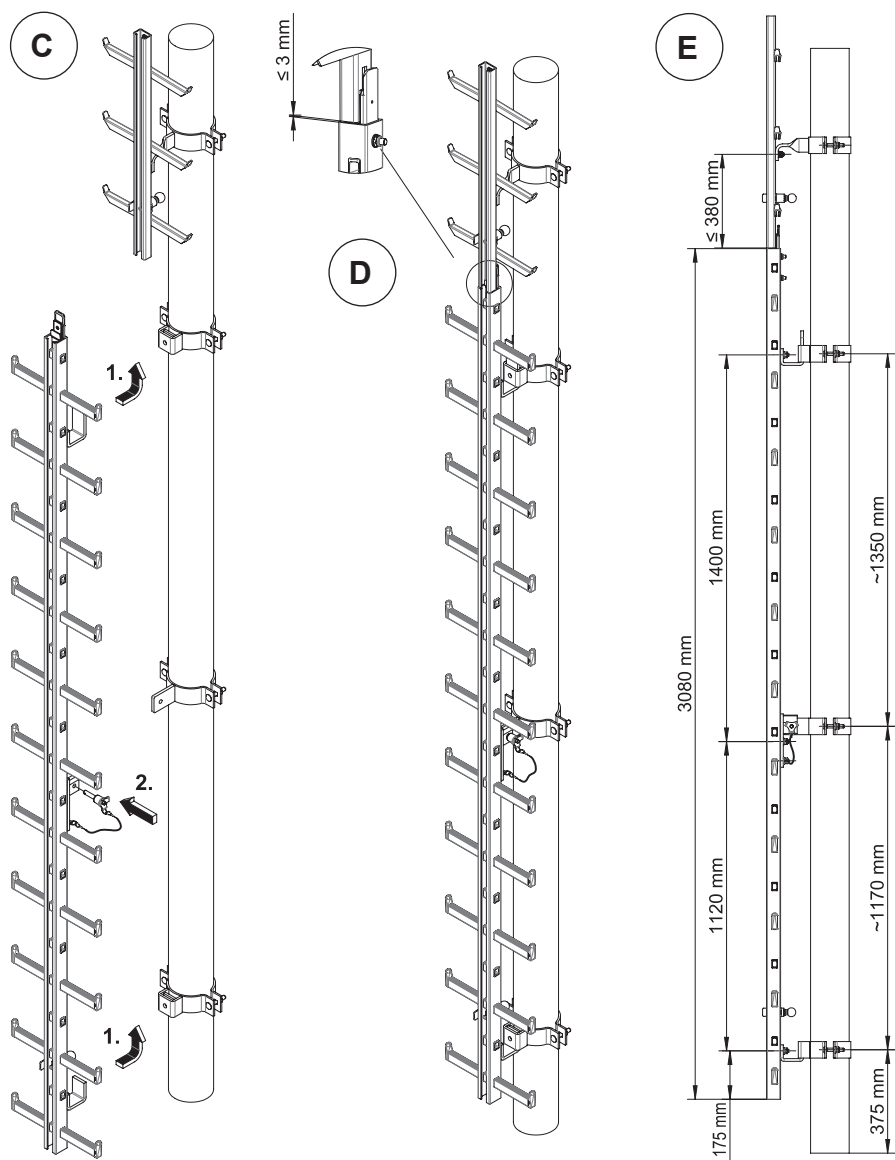
Obr. 2.18 - Zasouvací žebřík – montáž :
