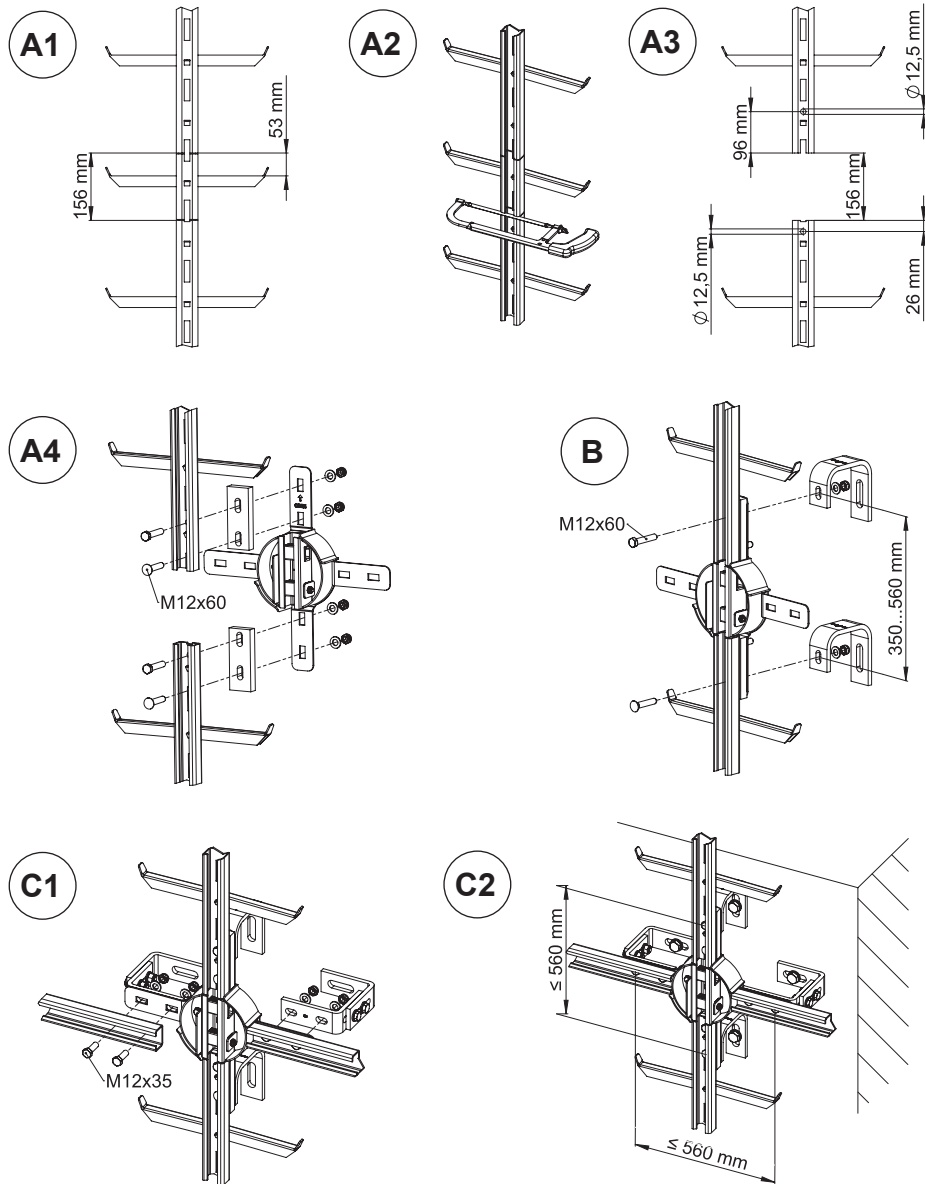
Obr. 2.12 - Točna se 4 konzolami - možnosti
