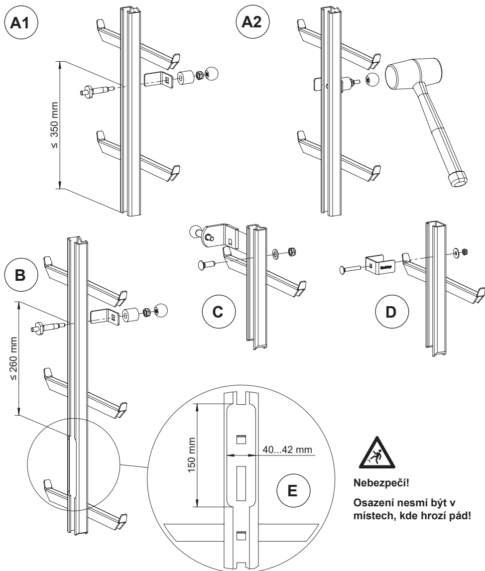
Obr. 2.2 - Instalace koncových zarážek
