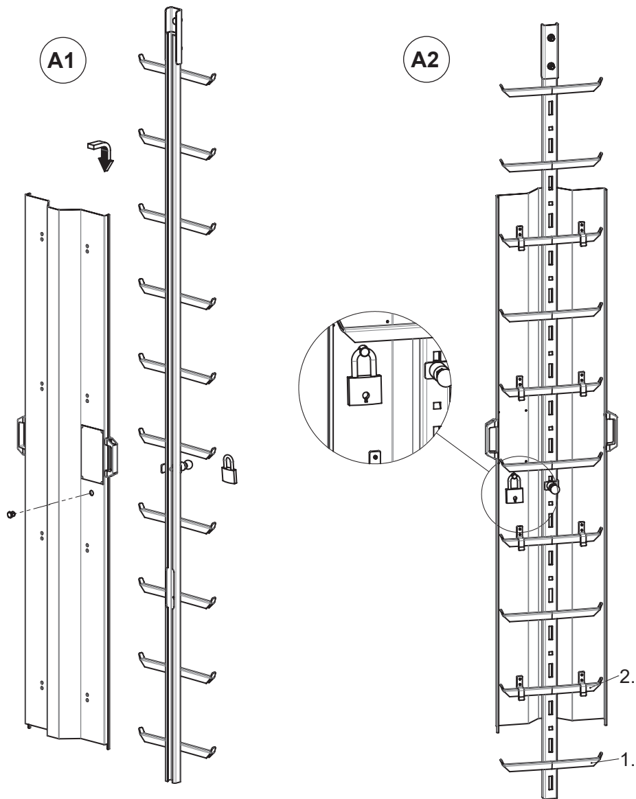
Fig. 2.7 - Krycí desky pro zavěšení, s držadly
