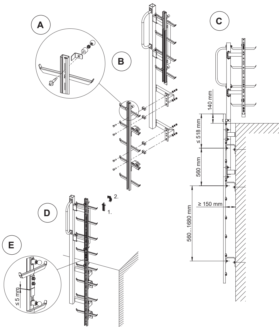
Obr. 2.11 - Otoč. střeš. výst.levý: A: Zarážka konstrukce B: Střešní výstup konstrukce C: Rozměry D: Provoz E: Max mezera v zajišt. režimu
