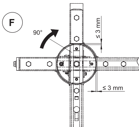
Obr. 2.13 - Točna se 4 konzolami - možnosti D1-D2: Instalace se 3 spoji (1 stop profil) E1-E2: Instalace se 2 spoji (2 stop profily) F: Provoz a rozměry mezer
