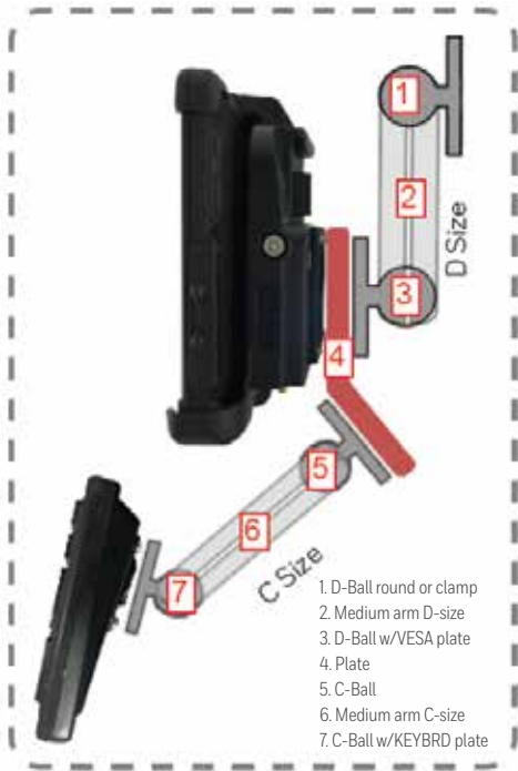
RT10-2015BRKTKIT
