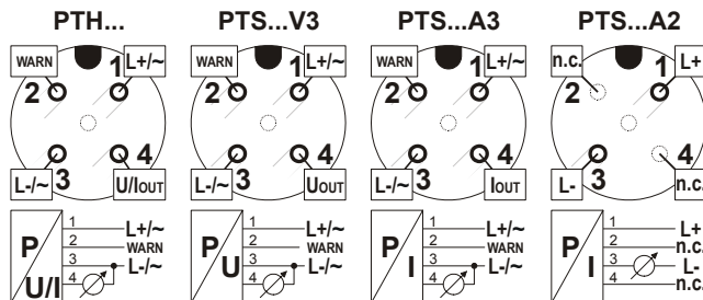
Abb. 3. A-codierter M12-Stecker
