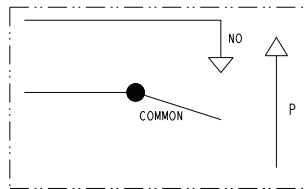
SPNO
