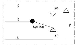
SPDT
