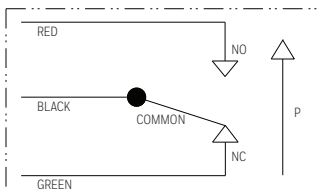
SPDT
